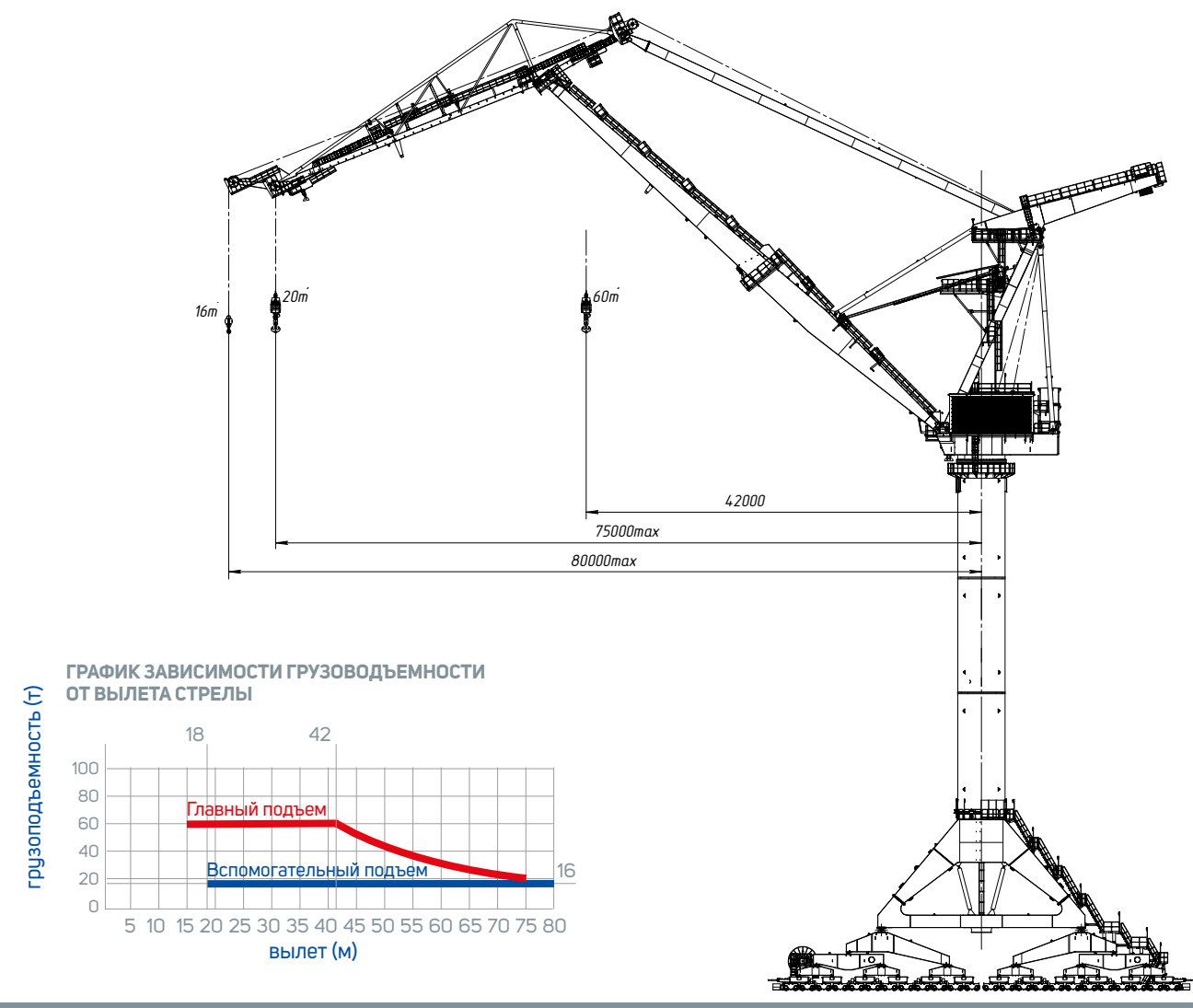
ЧЕРТЕЖ КРАНА СЕРИИ «СММ 2500»
