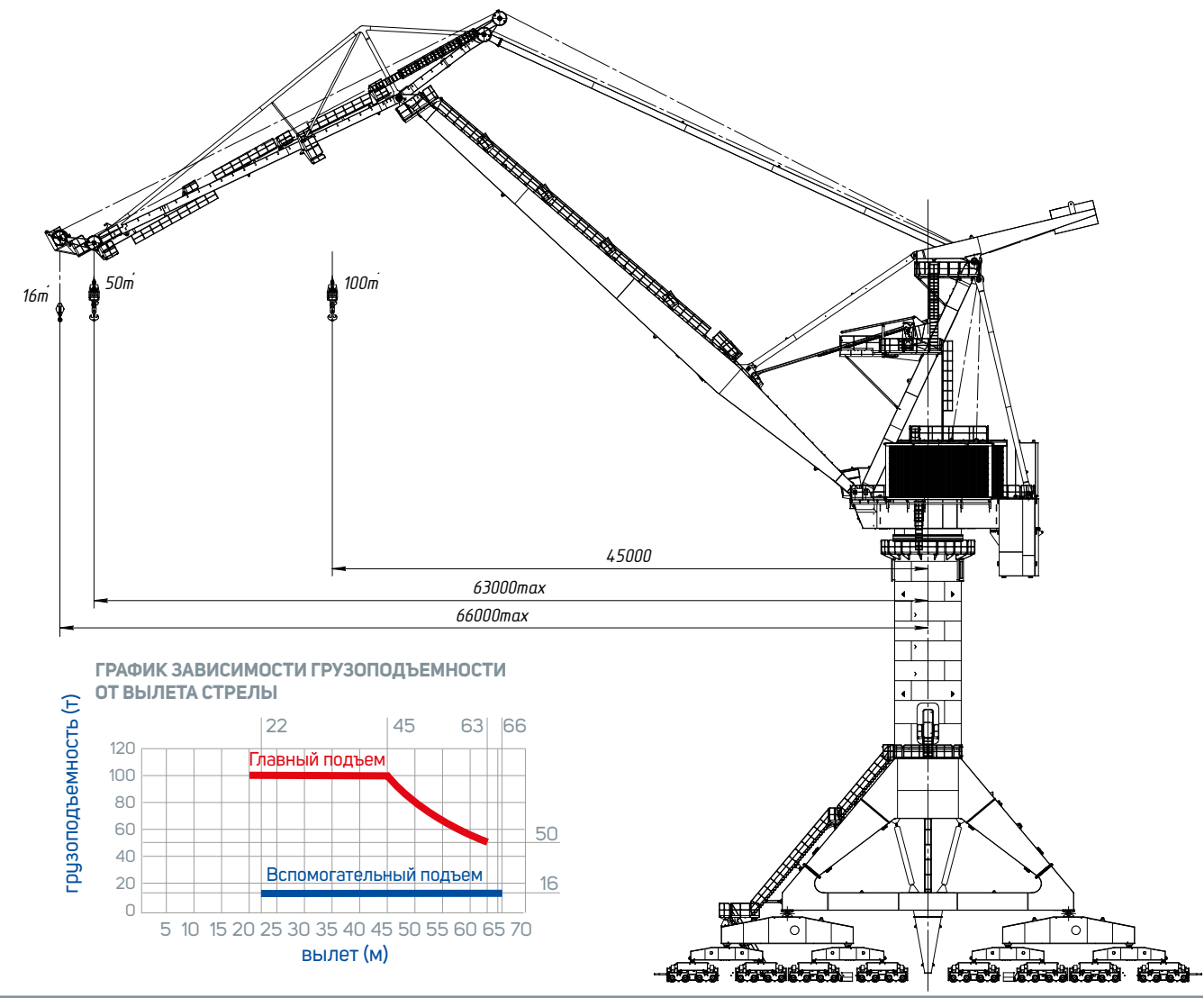
ЧЕРТЕЖ КРАНА СЕРИИ «СММ 4500»
