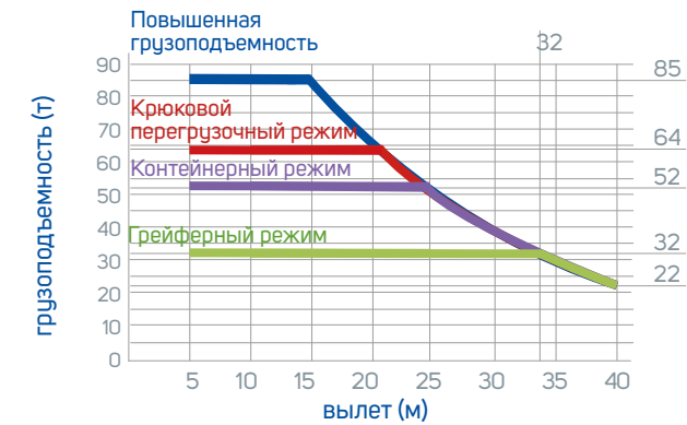
ГРАФИК ЗАВИСИМОСТИ ГРУЗОПОДЪЕМНОСТИ ОТ ВЫЛЕТА СТРЕЛЫ
