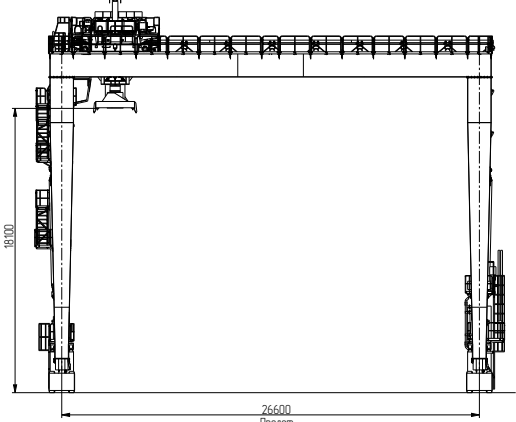
ЧЕРТЕЖ КРАНА СЕРИИ «БАРС-ПК»
