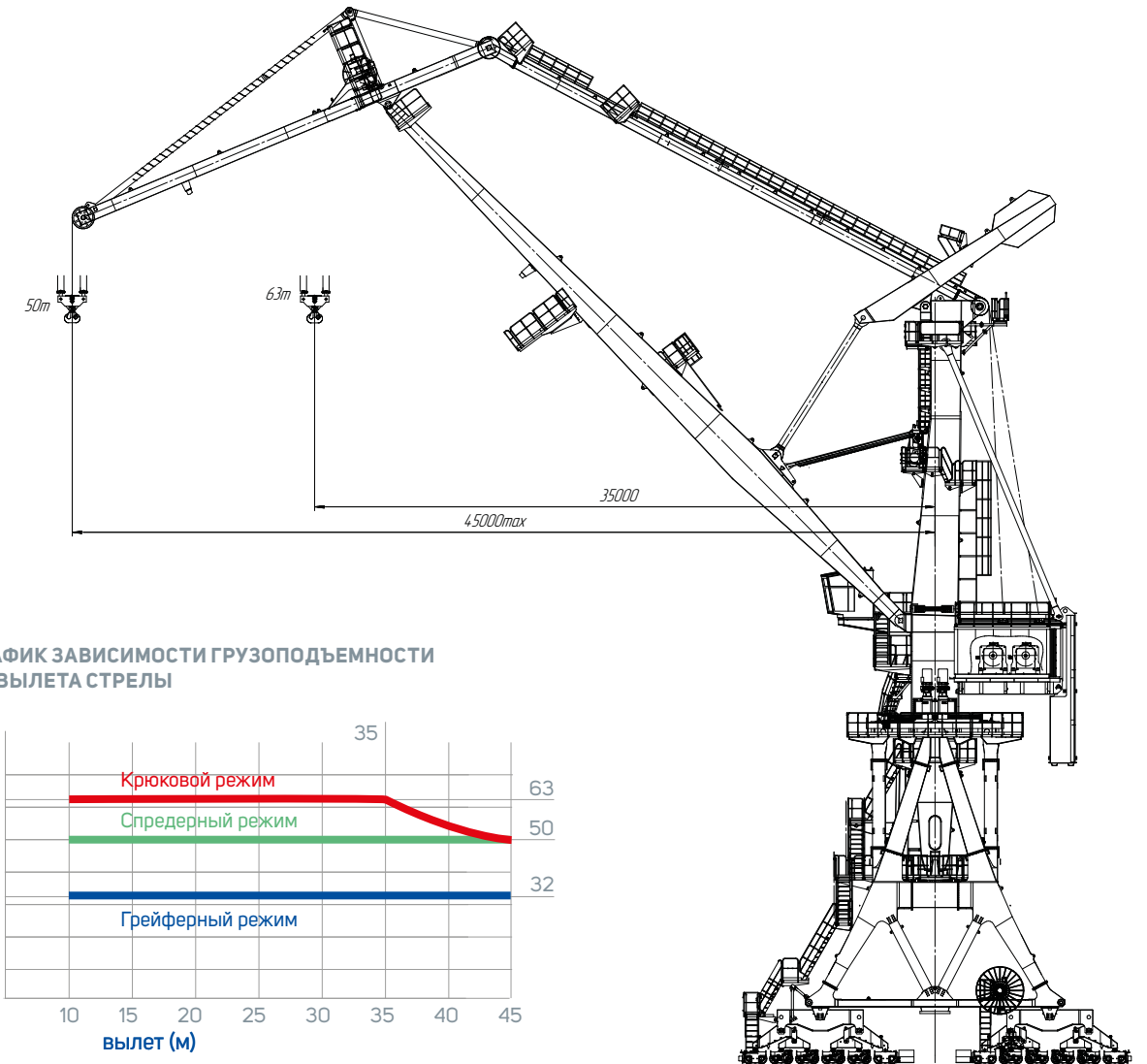
ЧЕРТЕЖ КРАНА СЕРИИ «ВИТЯЗЬ 2300»
