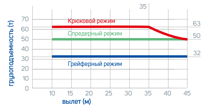
ГРАФИК ЗАВИСИМОСТИ ГРУЗОПОДЪЕМНОСТИ ОТ ВЫЛЕТА СТРЕЛЫ
