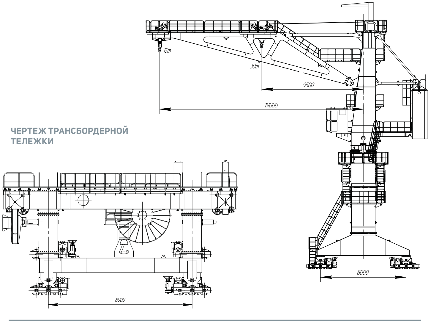
ЧЕРТЕЖ КРАНА СЕРИИ «СПК 3111»
