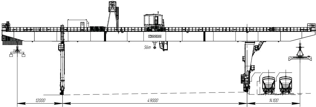
ЧЕРТЕЖ КРАНА СЕРИИ «БАРС»
