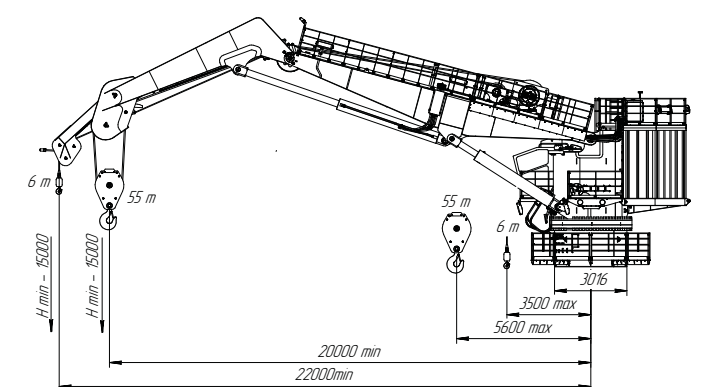
ЧЕРТЕЖ КРАНА СЕРИИ «КВ 1100»
