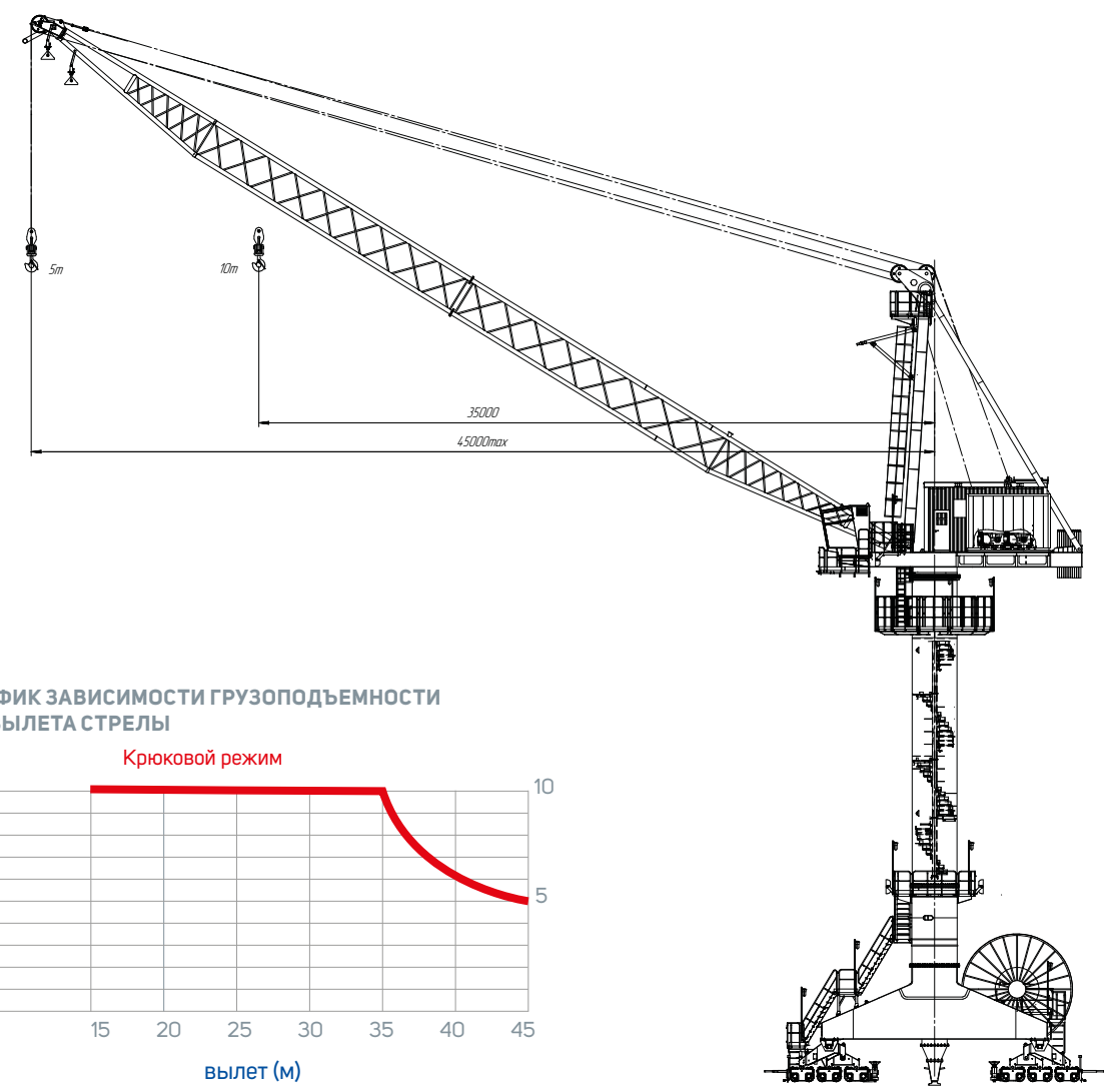
ЧЕРТЕЖ КРАНА СЕРИИ «ИБИС 350»
